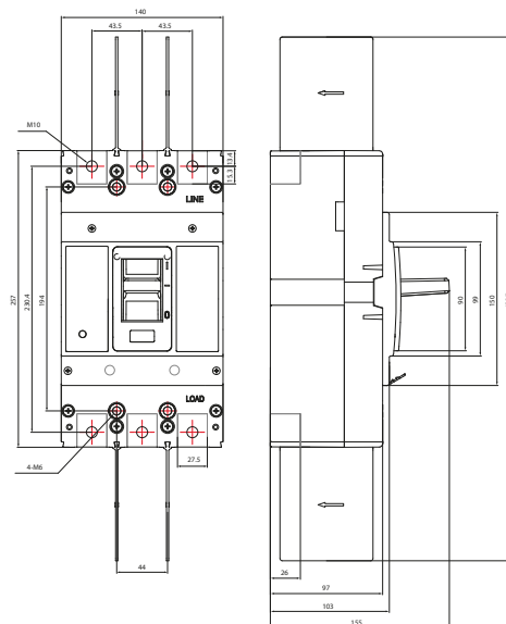
Méretrajz (AKM3,-4)
